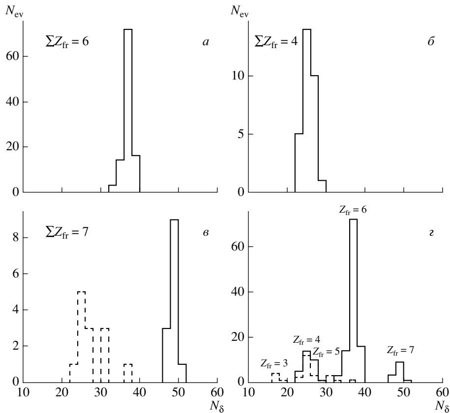
Рис. 2. Распределения числа N_{tr} следов пучковых частиц и вторичных фрагментов (штриховая гистограмма) по среднему числу \delta -электронов на 1 мм длины следа в “белых звездах” 2\text{He} + 2\text{H} (а), 2\text{He} и \text{He} + 2\text{H} (б) и в событиях с фрагментами Z_{fr} > 2 (в), а также распределение N_{tr} по N_{\delta} для всех измеренных событий (г).
