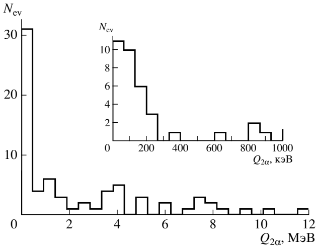
Рис. 3. Распределение числа “белых звезд” N_{ws} топологии 2\text{He} + 2\text{H} по энергии возбуждения Q_{2\alpha} пар \alpha -частиц; на вставке — увеличенное распределение Q_{2\alpha} .
