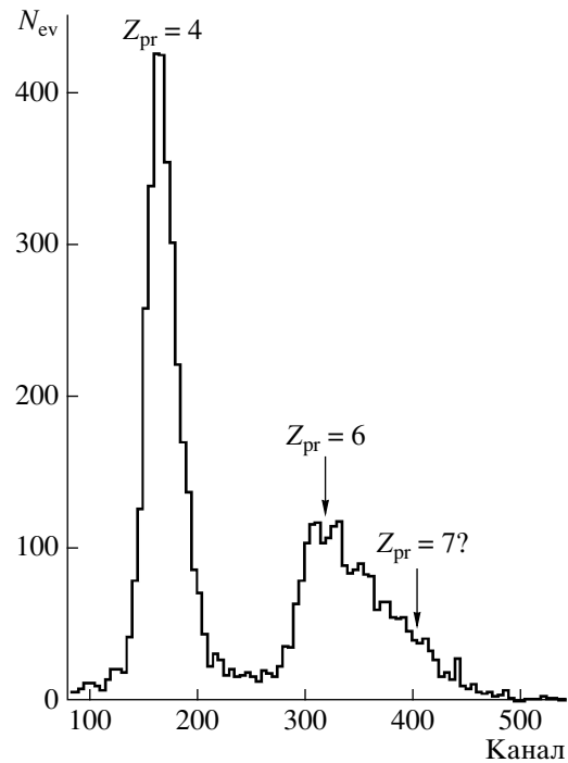
Рис. 1. Амплитудный спектр со сцинтилляционного счетчика, установленного на месте облучения эмульсионной стопки при настройке канала транспортировки пучка на сепарацию ядер ^{12}\text{N} ; указаны положения пиков для ядер с зарядами Z_{\text{pr}} = 4, 6 и 7 .
