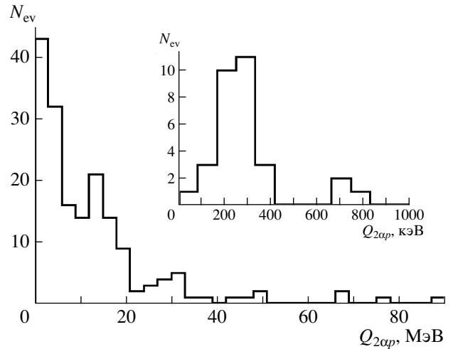
Рис. 4. Распределение числа “белых звезд” N_{ws} топологии 2\text{He} + 2\text{H} по энергии возбуждения Q_{2\alpha p} троек 2\alpha + p ; на вставке — увеличенное распределение Q_{2\alpha p} .
